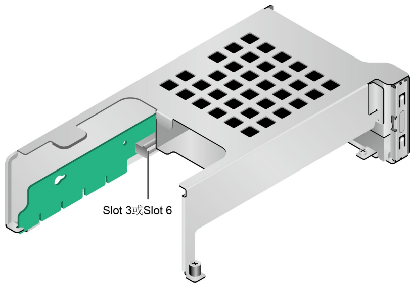
图 5-29 1x16 Riser 卡
