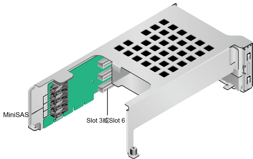
图 5-30 SAS Riser 卡
