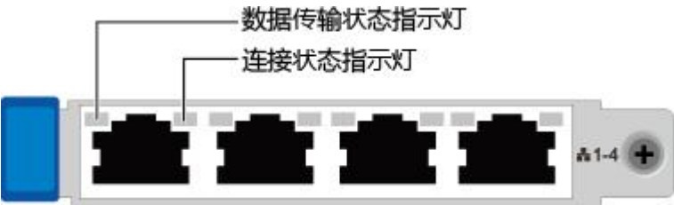
图 5-12 TM210/TM211（4*GE 电口）
