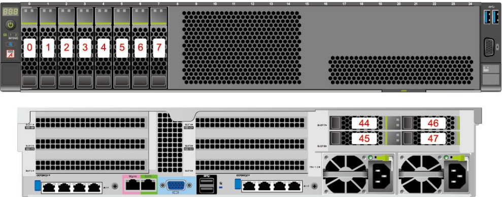
图 5-18 8x2.5 英寸硬盘配置的硬盘编号
