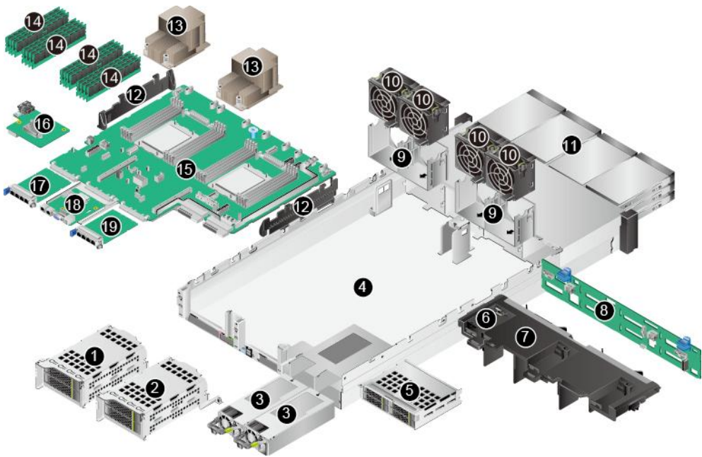
图 3-2 部件（配置鲲鹏 920 5220、3210 或 5225F 处理器）
