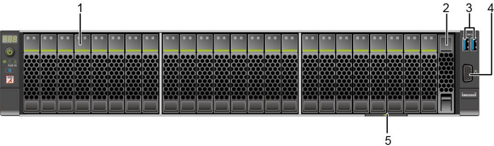
图 5-3 24x2.5 SAS/SATA 直通硬盘配置前面板组件
