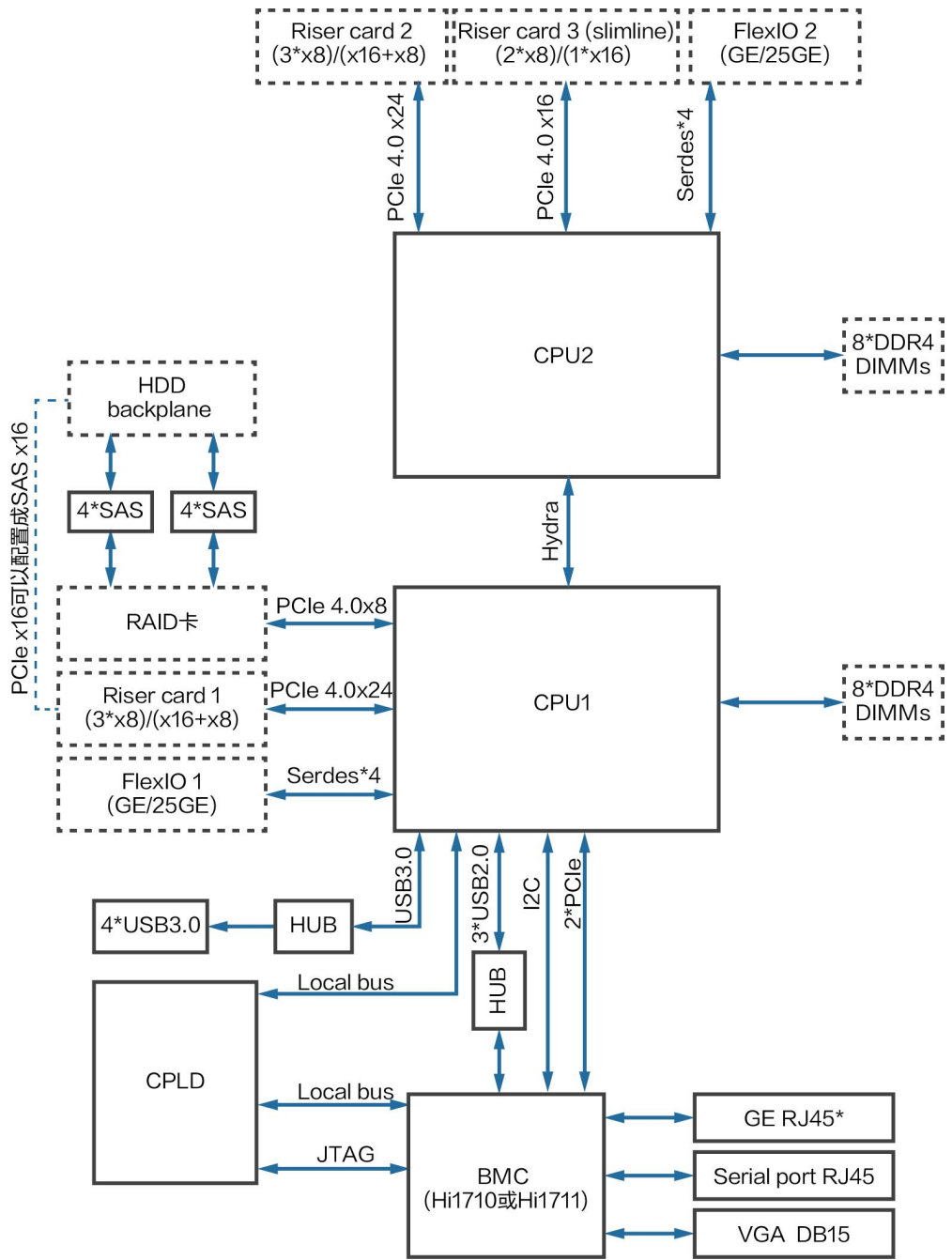
图 4-2 服务器逻辑结构（配置鲲鹏 920 5220、3210 或 5255F 处理器）
