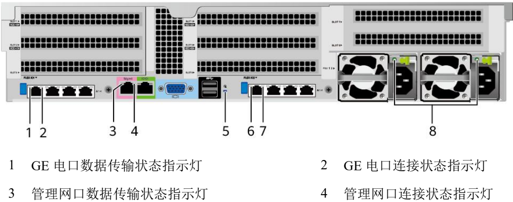
图 5-11 后面板指示灯
