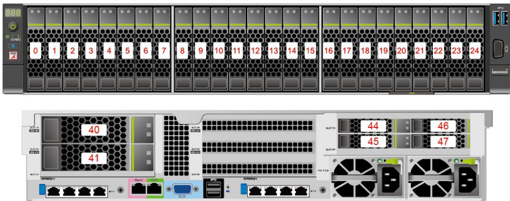
图 5-16 25x2.5 英寸硬盘 EXP 配置硬盘编号
