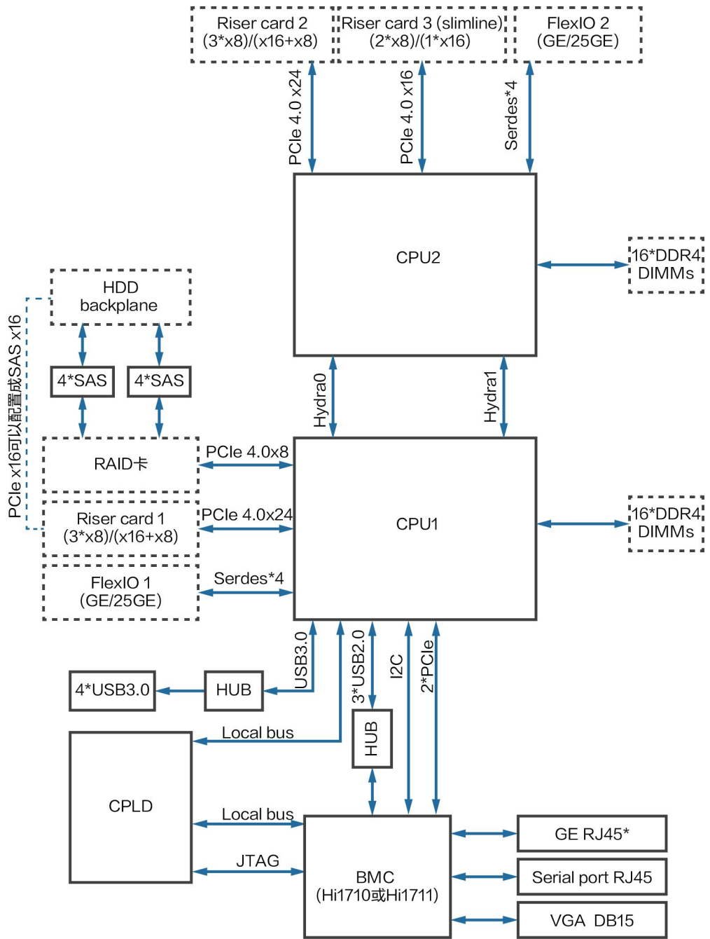
图 4-1 服务器逻辑结构（配置鲲鹏 920 7260、5250、7265F 或 5255F 处理器）
