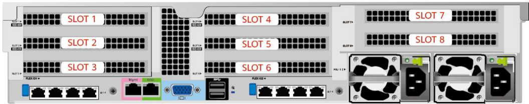
图 5-24 PCIe 插槽
