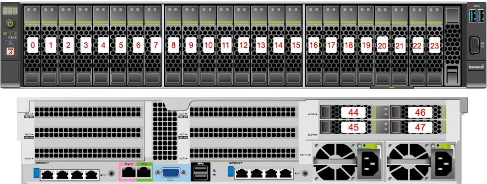
图 5-17 24x2.5 SAS/SATA 硬盘直通配置
