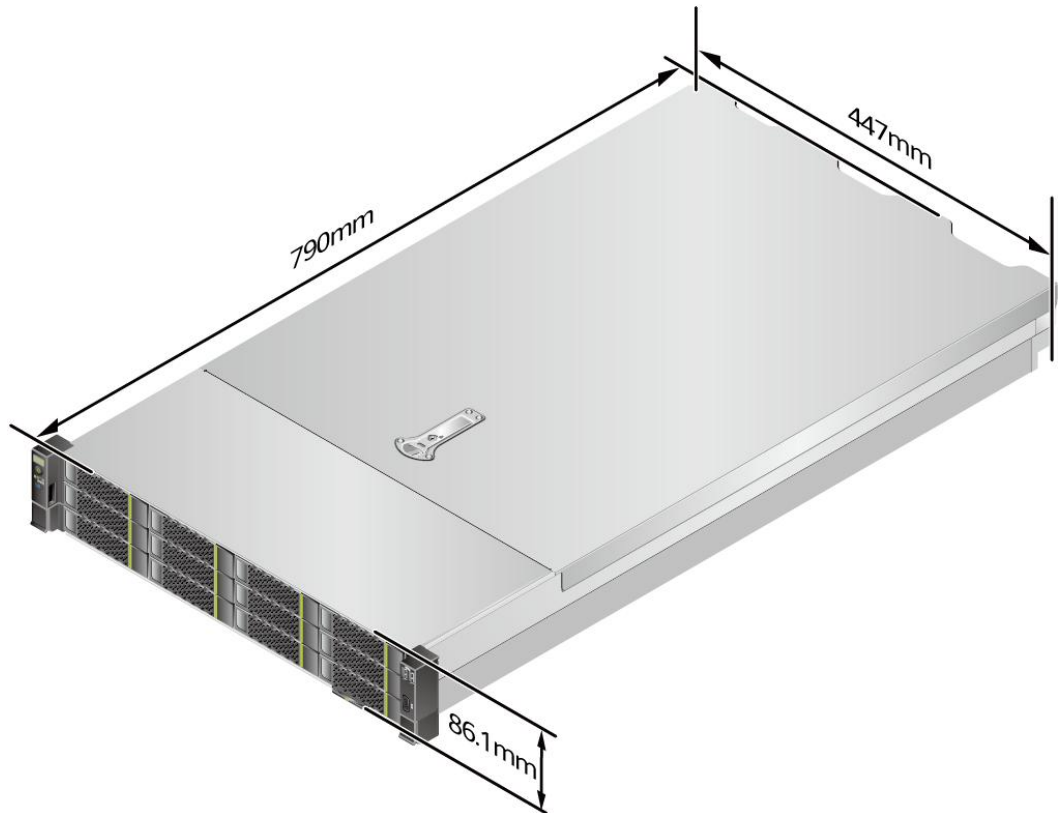
图 6-2 物理尺寸
