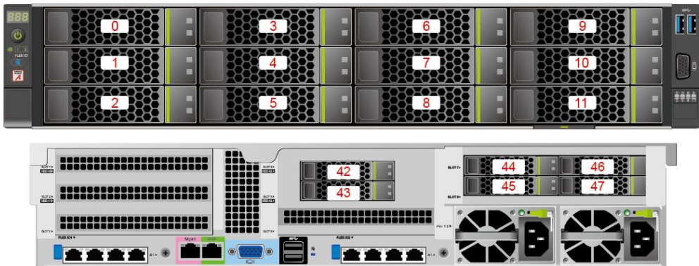
图 5-15 12x3.5 英寸硬盘直通配置
