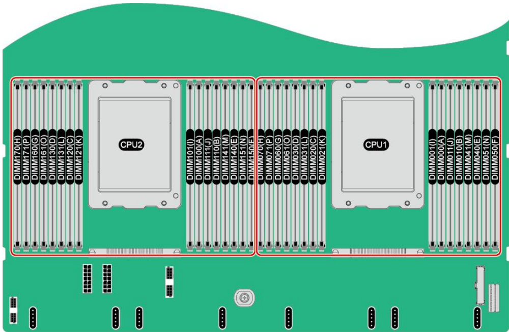
图 5-22 内存槽位编号（配置鲲鹏 920 7260、5250、7265F 或 5255F 处理器）
