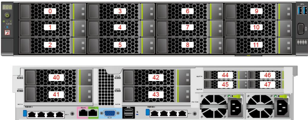
图 5-14 12x3.5 英寸硬盘 EXP 配置硬盘编号
