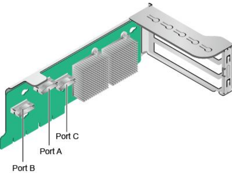
图 5-28 12NVMe 专用 Riser 卡
