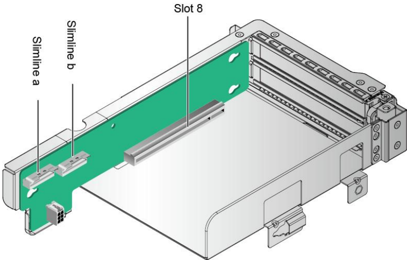
图 5-32 1x16 Riser 卡
