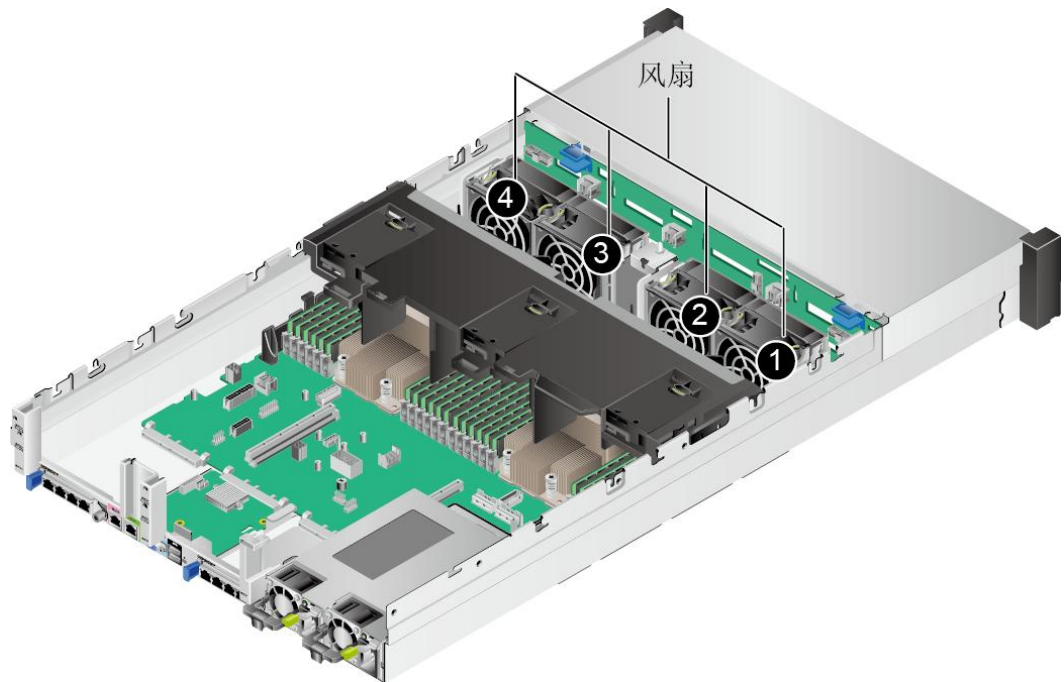
图 5-33 风扇位置示意图
