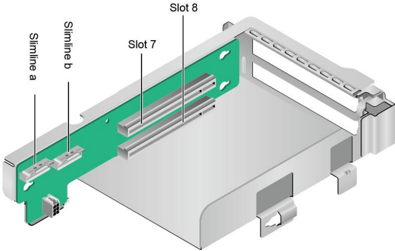
图 5-31 2x8 Riser 卡
