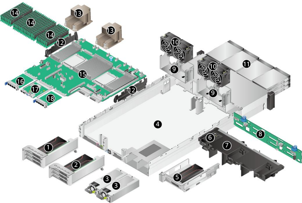
图 3-1 部件（配置鲲鹏 920 7260、5250、7265F 或 5255F 处理器）
