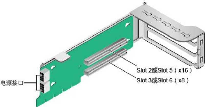
图 5-27 1x8+1x16 Riser 卡
