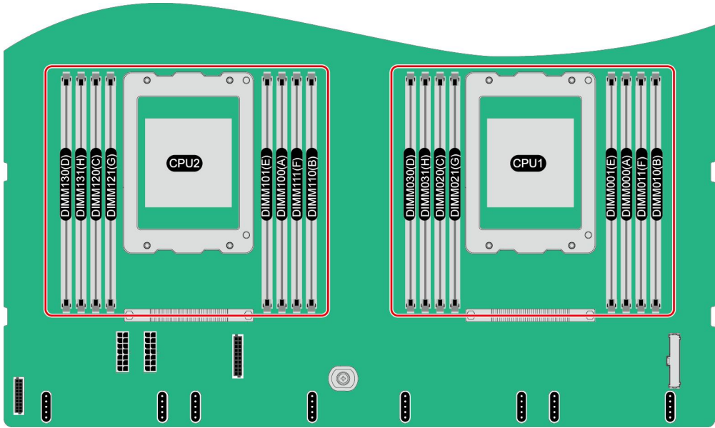
图 5-23 内存槽位编号（配置鲲鹏 920 5220、3210 或 5225F 处理器）
