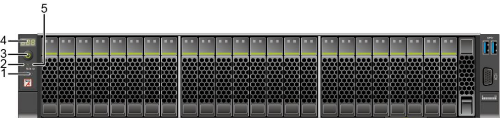
图 5-8 24x2.5 SAS/SATA 直通硬盘配置前面板指示灯和按钮
