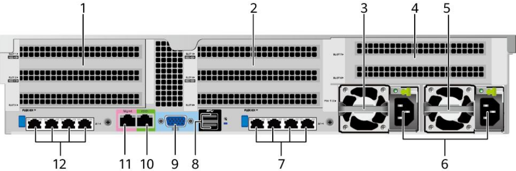
图 5-10 后面板组件
