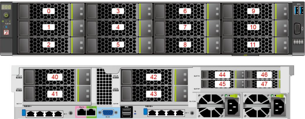
图 5-19 12x3.5 英寸硬盘 RAID 直通配置编号
