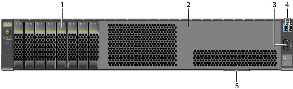
图 5-4 8x2.5 英寸硬盘配置前面板组件
