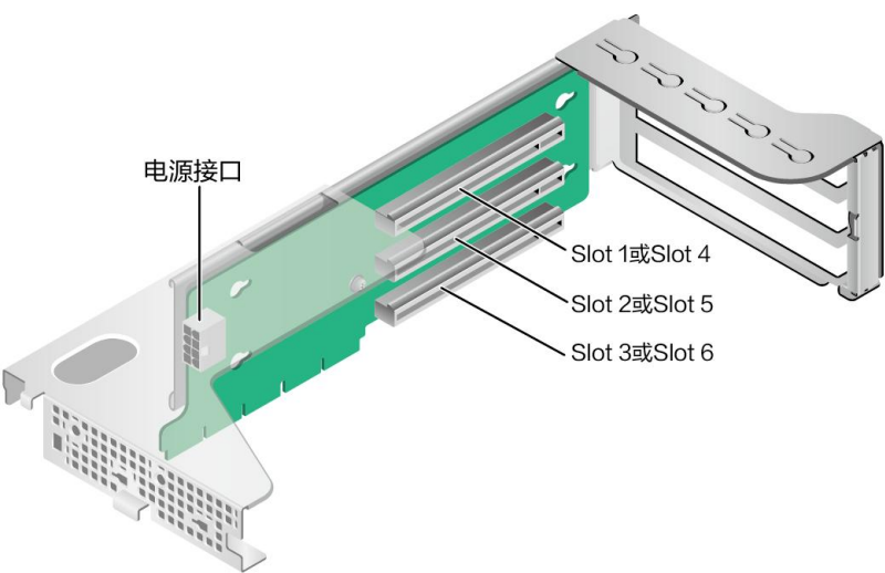
图 5-26 3x8 Riser 卡
